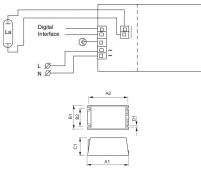
Caractéristiques Philips HID-DV PROG Xt 250 SON C2 208-277V for 250W
